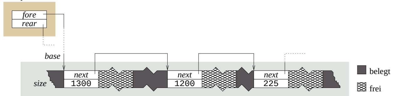
Freispeicherliste
